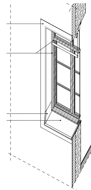
Détail menuiserie avec store
