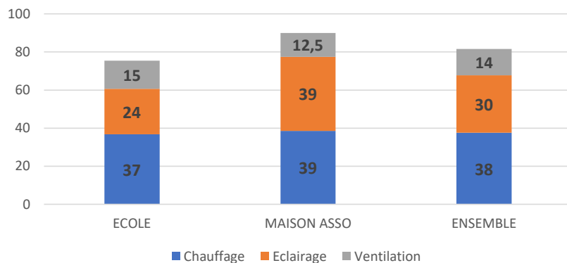
Consommations conventionnelles RTEx (kWh ep /m 2 /an)
