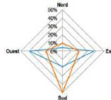
REPARTITION DES VITRAGES MAISON DES ASSOCIATIONS
