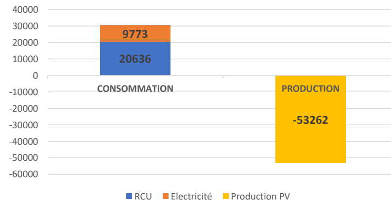
Consommations et production finale (kWh ep )
