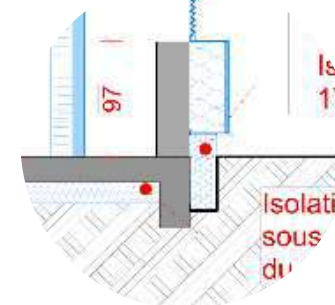
Liaison sol-mur
